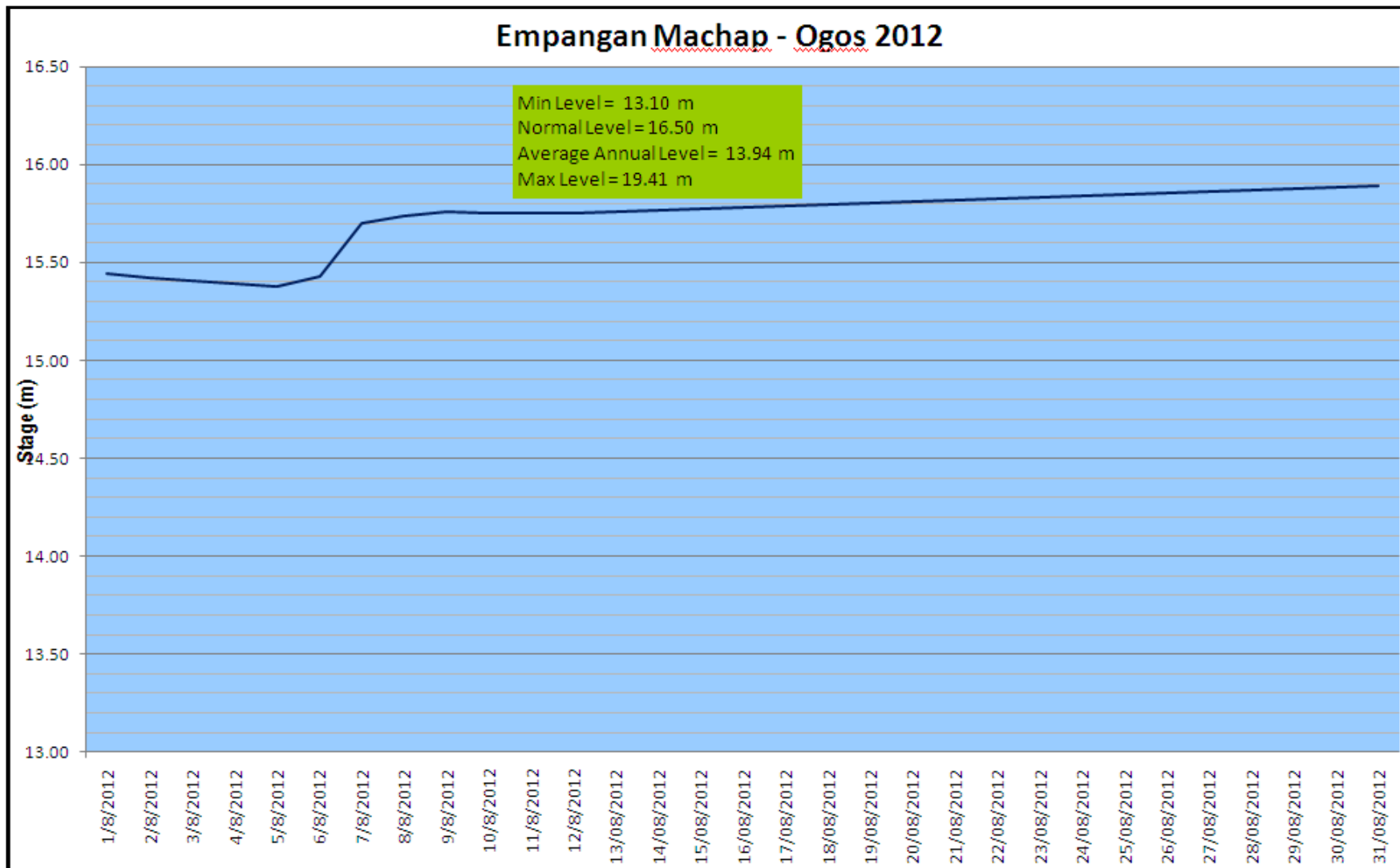
Rajah 6 (i) : Rekod Aras Empangan Machap, Johor pada bulan Ogos 2012
