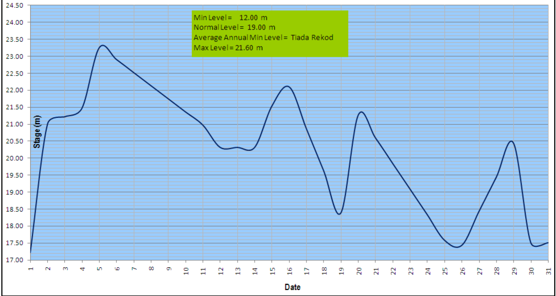
Rajah 6 (vi) : Rekod Aras Empangan Anak Endau, Pahang pada bulan Ogos 2012
