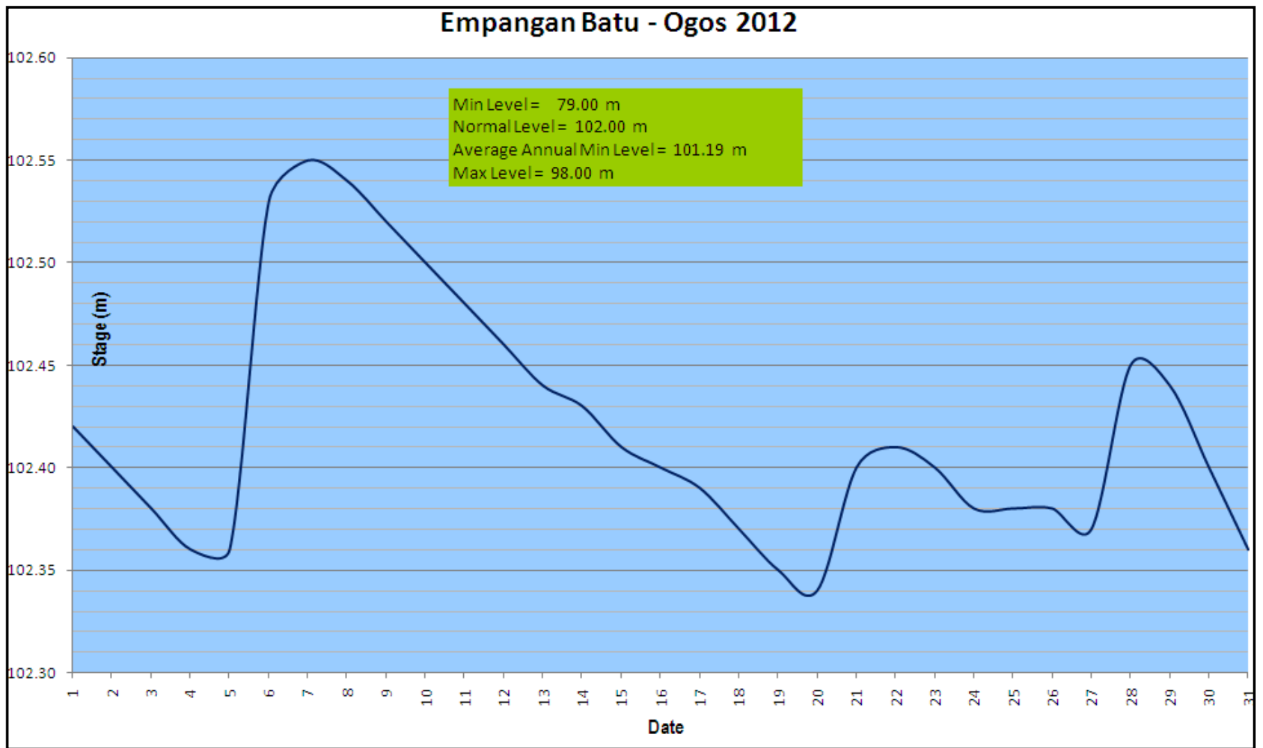
Rajah 6 (ix) : Rekod Aras Empangan Batu, KL pada bulan Ogos 2012
