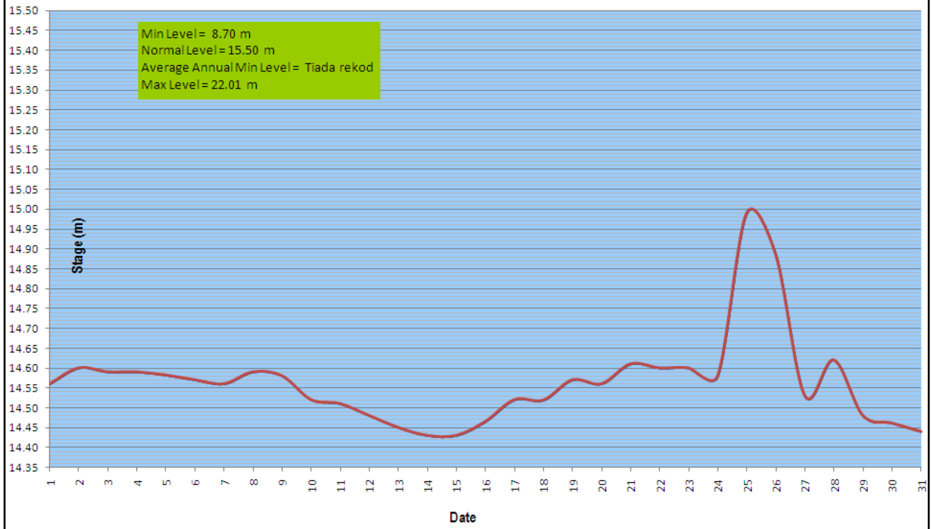
Rajah 6 (iii) : Rekod Aras Empangan Bekok, Johor pada bulan Ogos 2012
