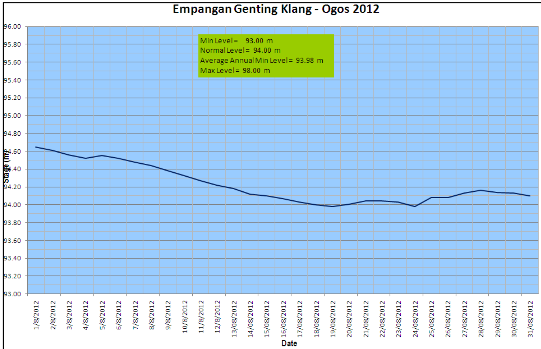
Rajah 6 (x) : Rekod Aras Empangan Genting Kelang, KL pada bulan Ogos 2012
