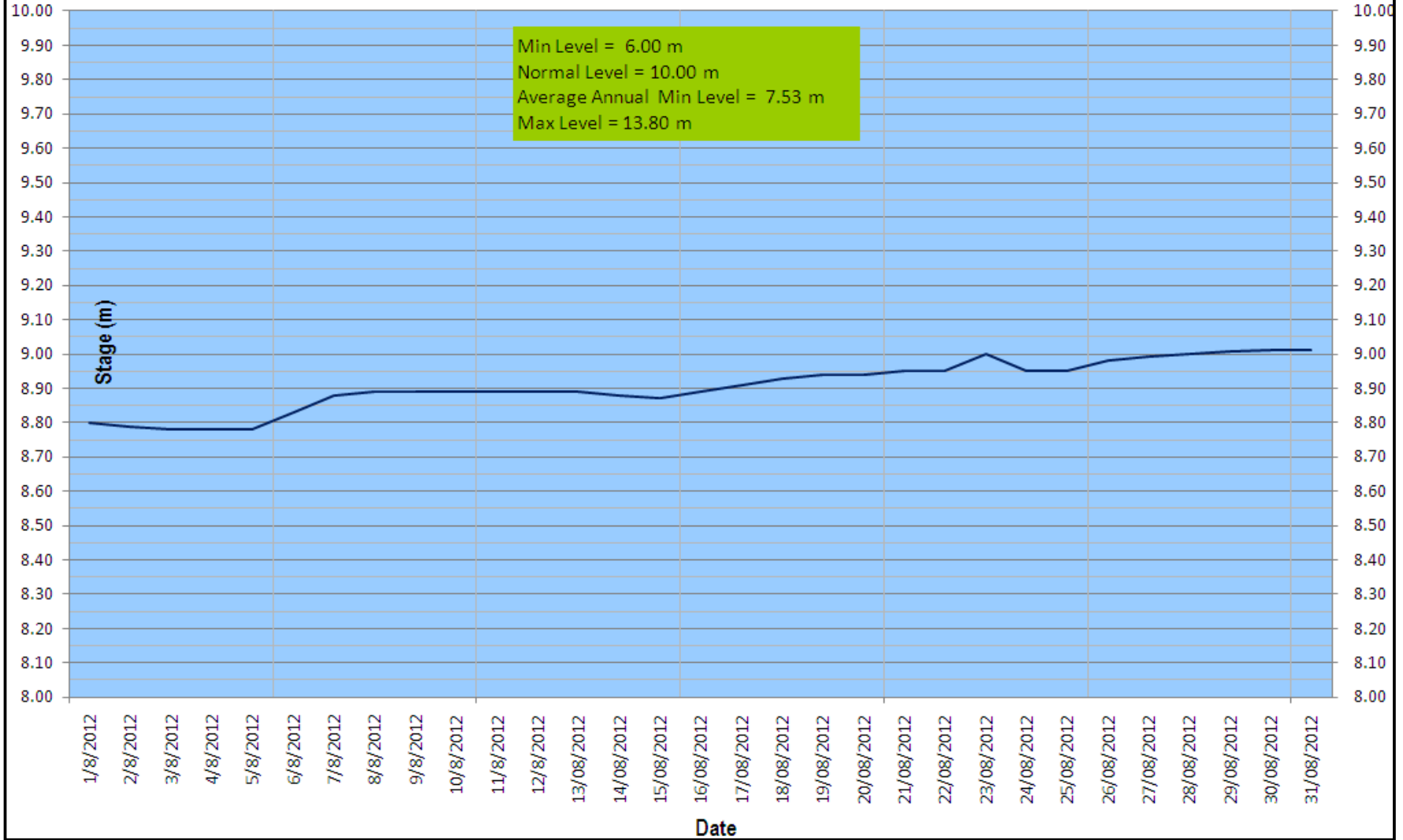
Rajah 6 (ii) : Rekod Aras Empangan Sembrong, Johor pada bulan Ogos 2012
