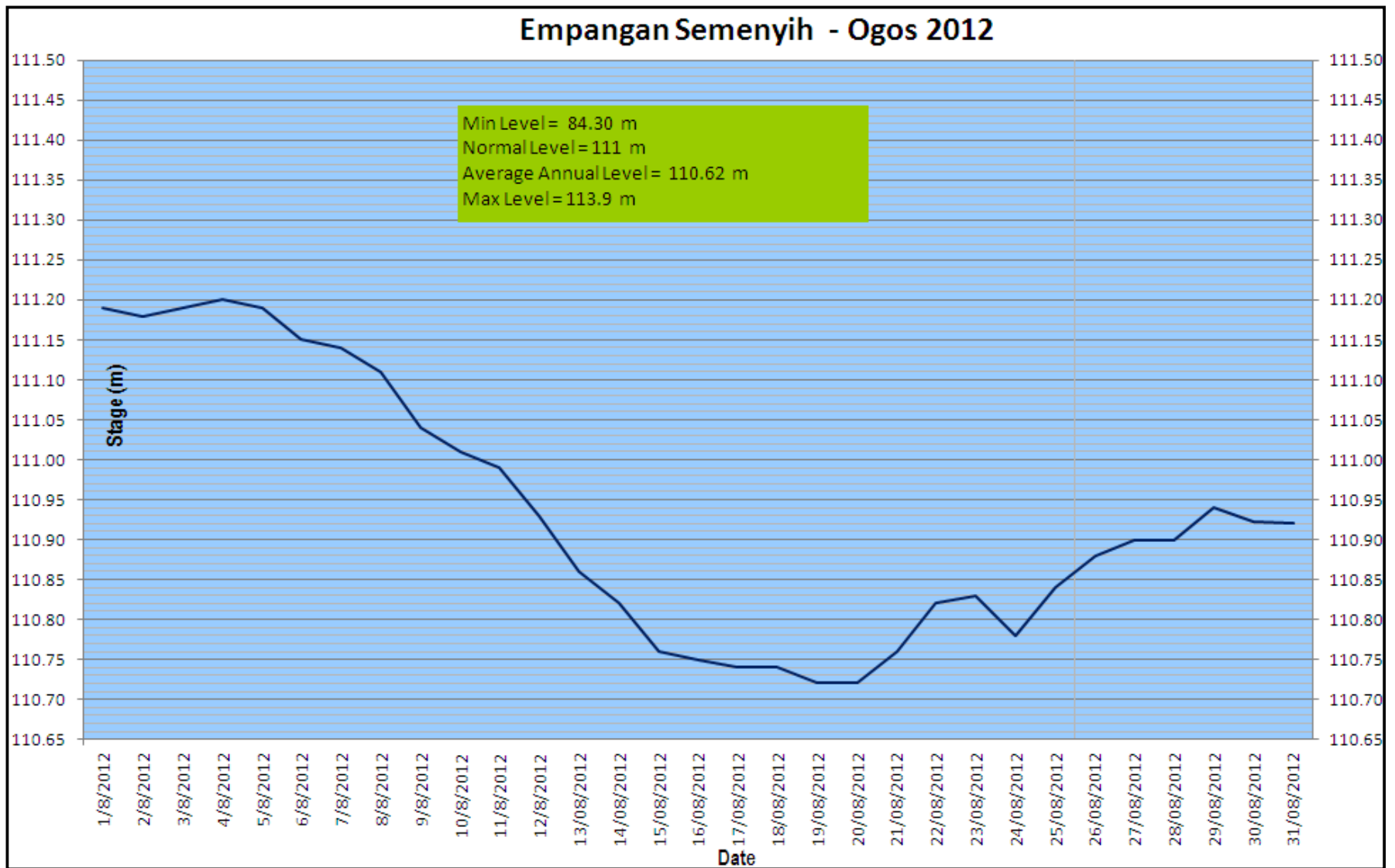
Rajah 6 (viii) : Rekod Aras Empangan Semenyih, Selangor pada bulan Ogos 2012
