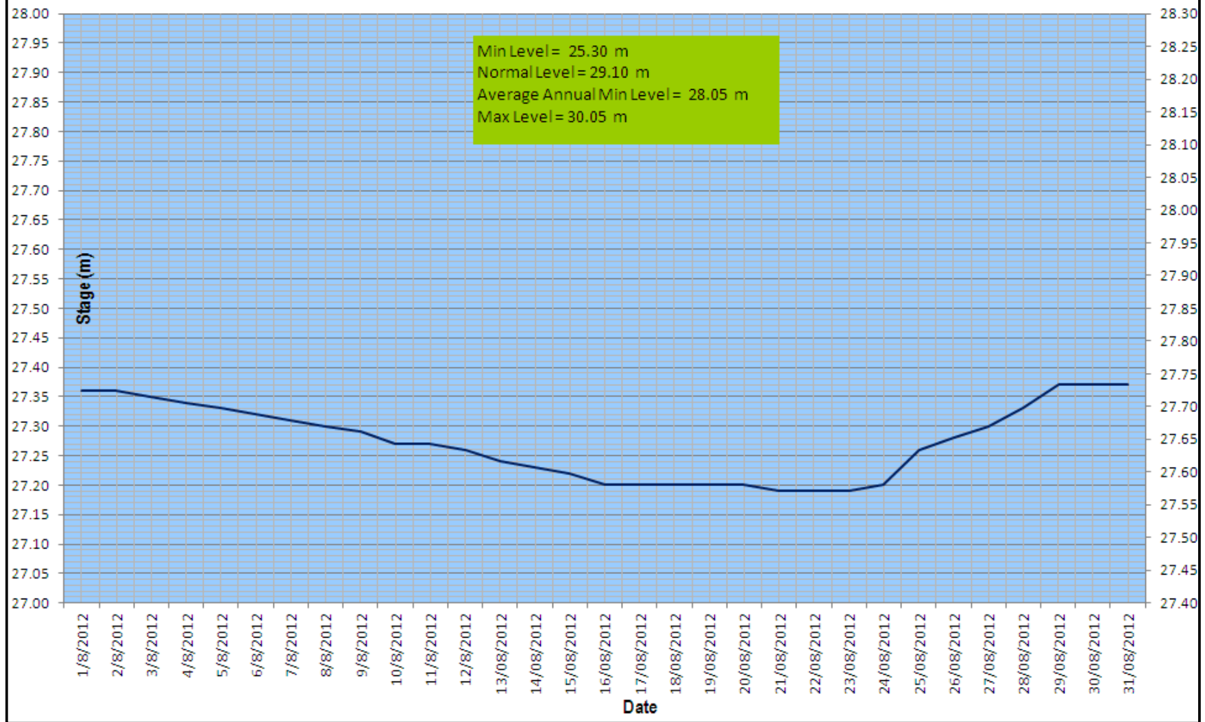
Rajah 6 (vii) : Rekod Aras Empangan Timah tasoh, Perlis pada bulan Ogos 2012
