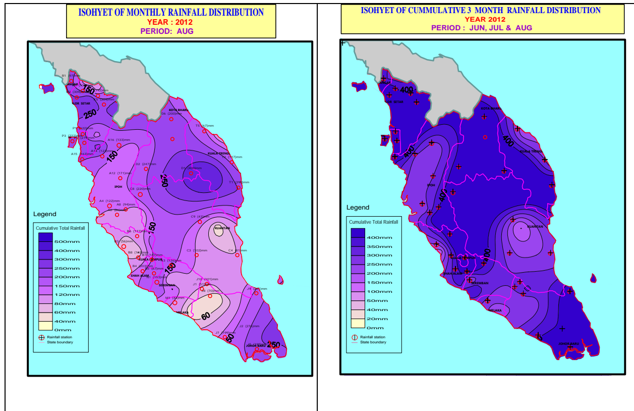
Rajah 2: Taburan Hujan Bulan Ogos
