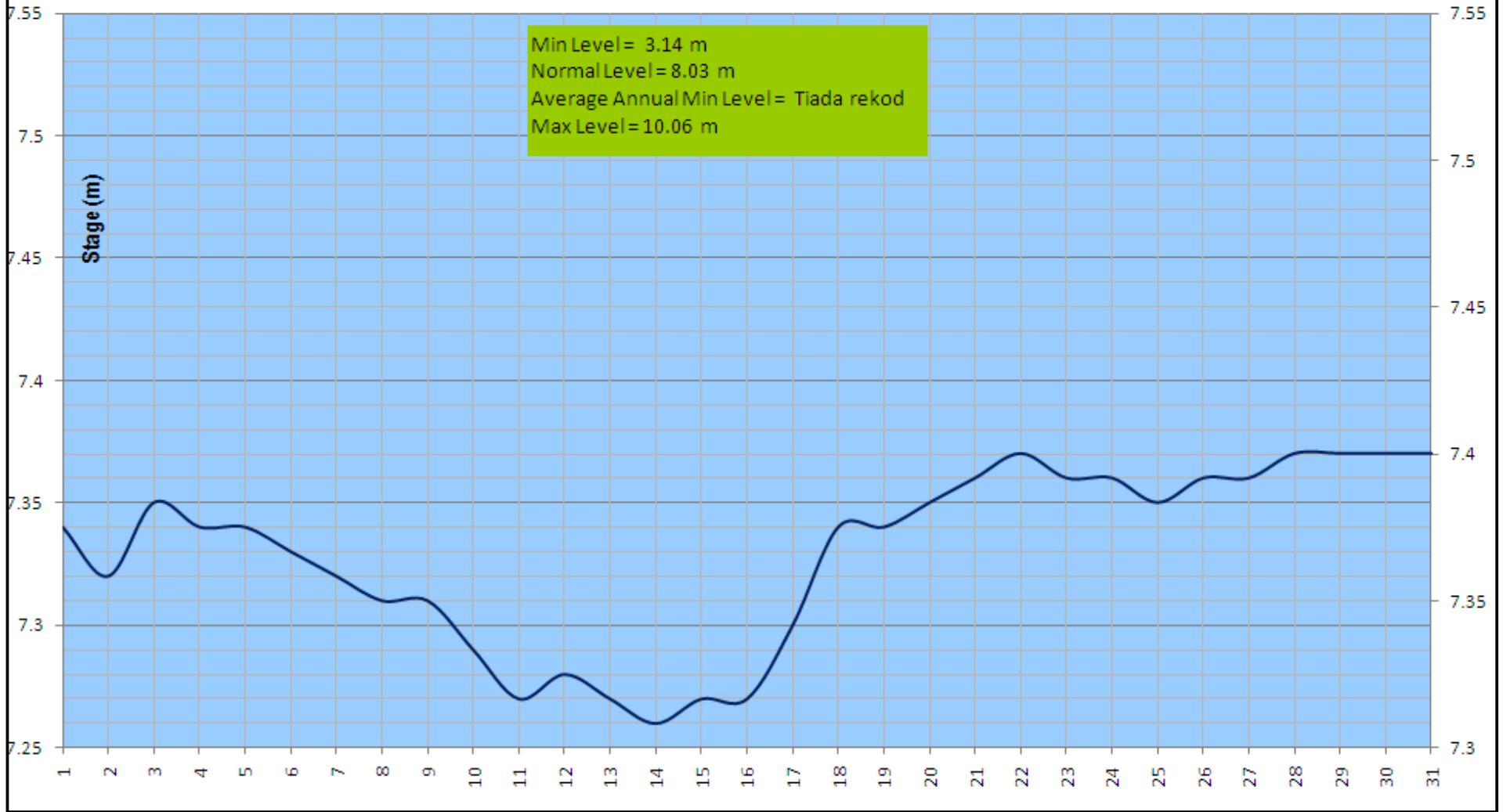
Rajah 6 (iv) : Rekod Aras Empangan Labong, Johor pada bulan Ogos 2012
